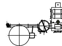
KOMORA PRIPOJENA KE KOTLI Z LEVA
